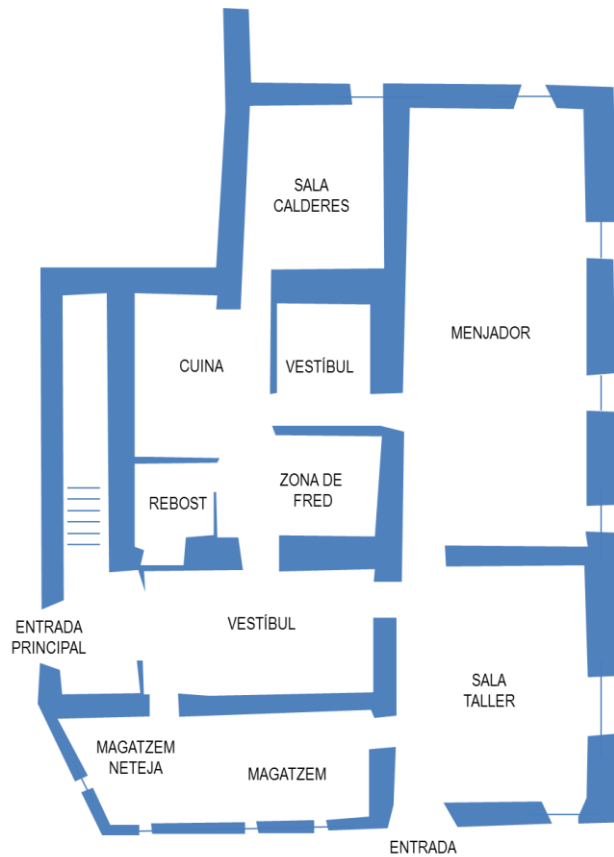
PLANTA BAIXA
